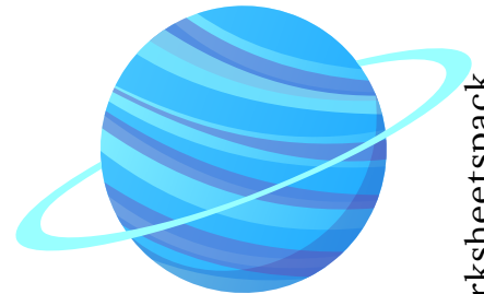
Uranus
